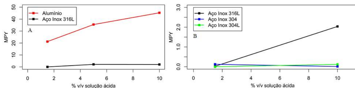
Figura 1 – Comparação da corrosão das amostras.
