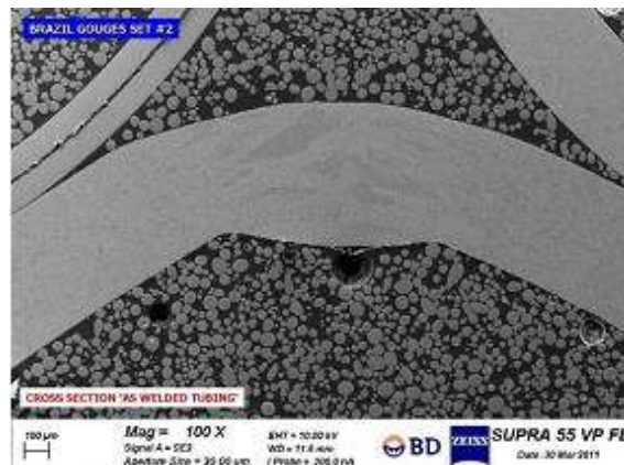
Figura 7. Detalhe da microestrutura do cordão de solda através da microscopia.
